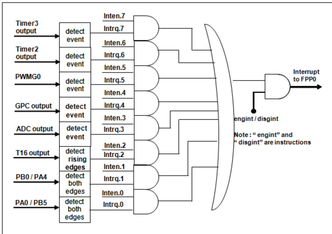
图 13: 中断硬件框图
