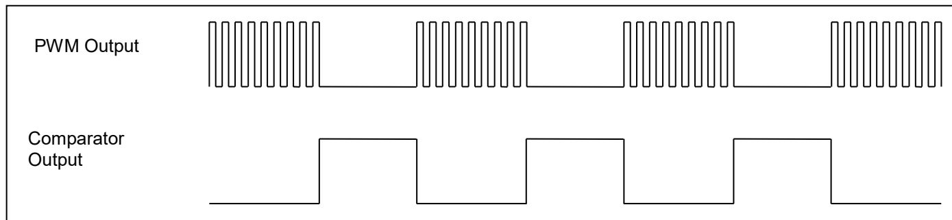
图 18: 比较器控制 PWM 输出
