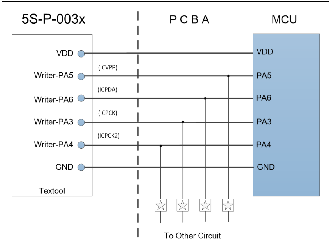
图 32: 在板烧录接线示意图
